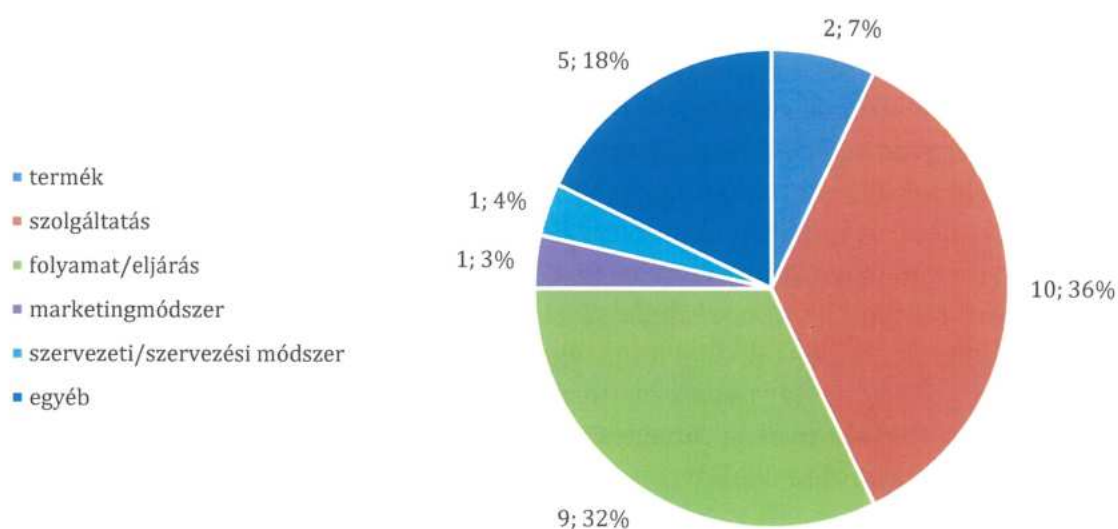
Innovációtípusok megoszlása 2023
